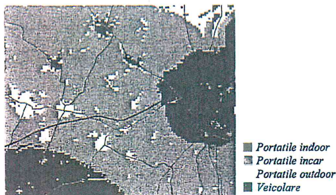
Figura 6 - Esempio di mappa di copertura radioelettrica.
